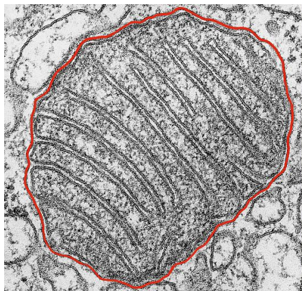
Slika 116. Mitohondrija (TEM)
