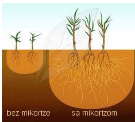
Slika 148. Mikoriza - desno
