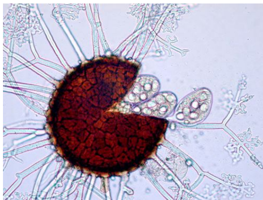
Slika 185. Kleistotecijum
