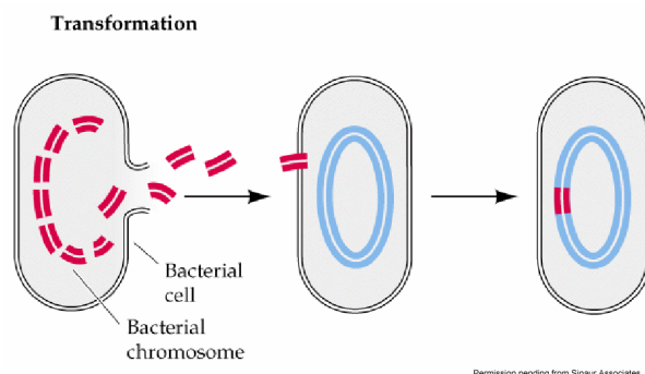
Slika 191. Transformacija
