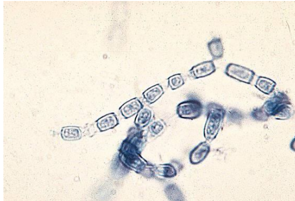
Slika 179. Artrospore
