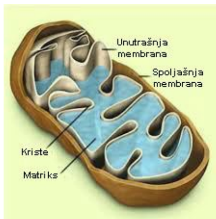
Slika 115. Šematski prikaz građe mitohondrije
